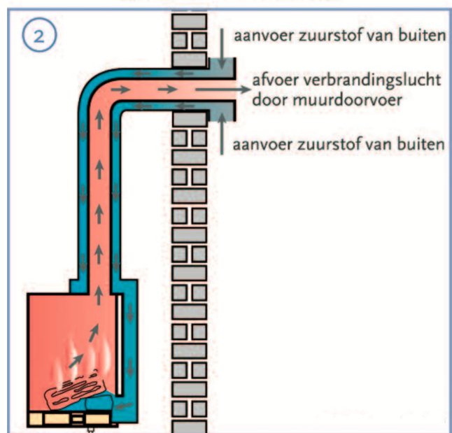
'gesloten' verbranding
