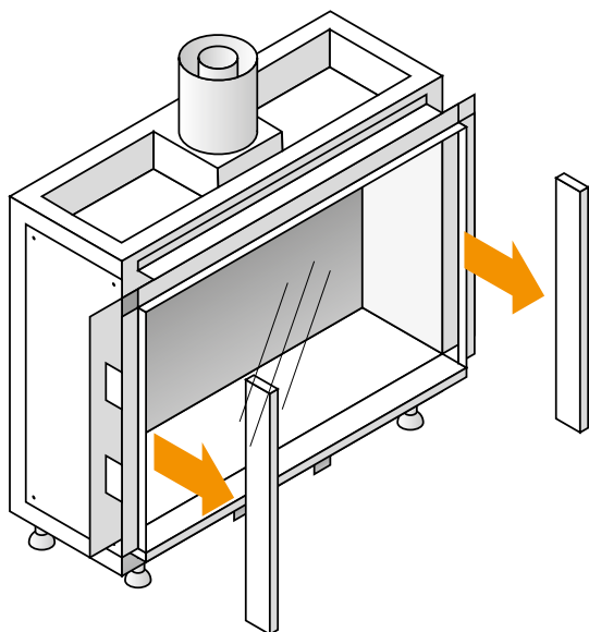
Afbeelding 10-2: Verwijderen van de zijlijsten
