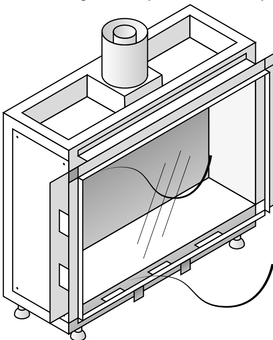
Afbeelding 10-4: Verwijderen van de koorden
