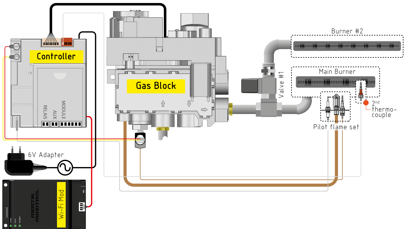
Afbeelding 9-1: Aansluitschema Modore 75H
