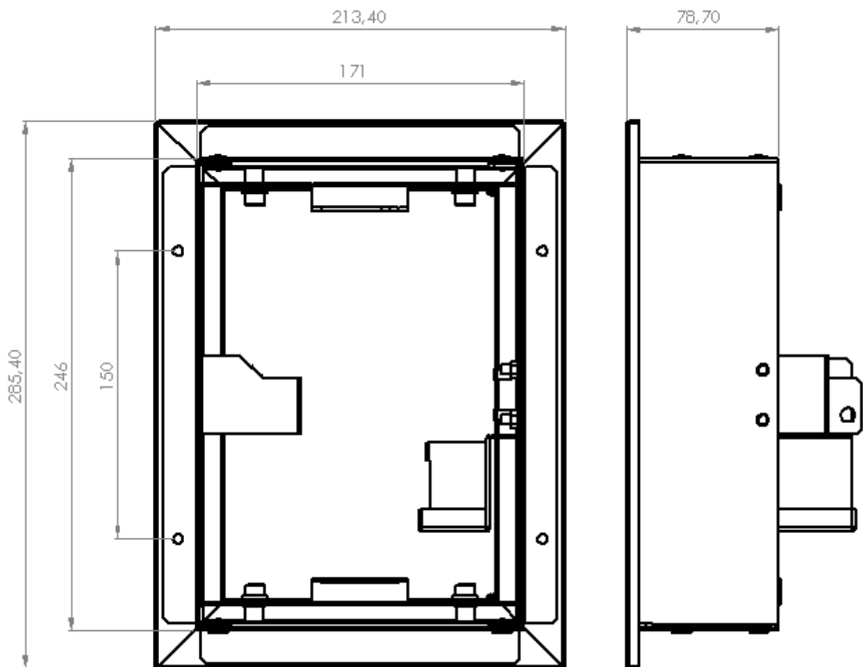
Afbeelding I-1: Bedieningsluik, BDLE4
