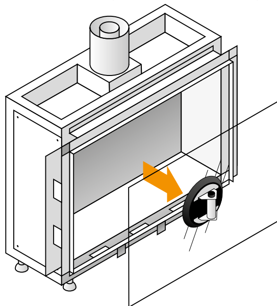
Afbeelding 10-6: Uithalen van het glas
