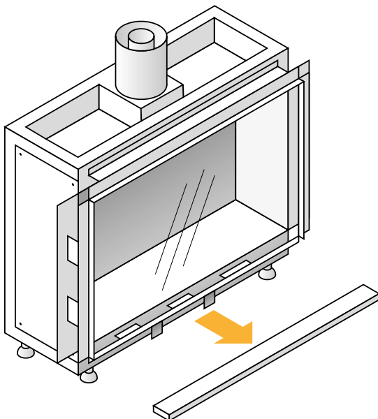
Afbeelding 10-3: Verwijderen van de onderlijst
